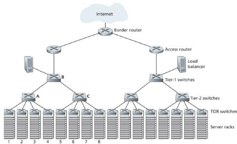
شکل ۲: Hierarchical data center network
